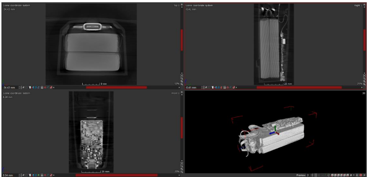
Fig. 16 – Images aux rayons X de la batterie d'ANAFI Thermal
