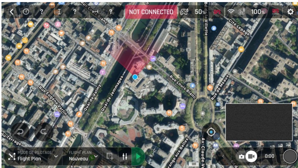
Fig. 11 : Cartographie iOS
