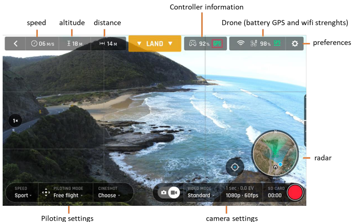
Fig. 9 : Interface FreeFlight 6
