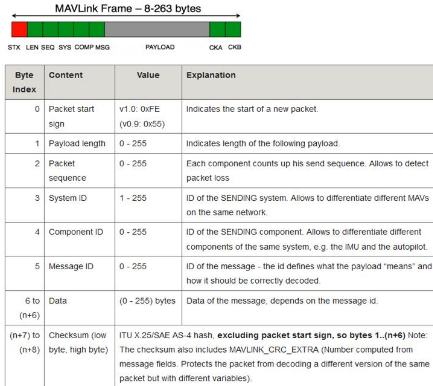
Fig. 14 : Protocole MAVLink
